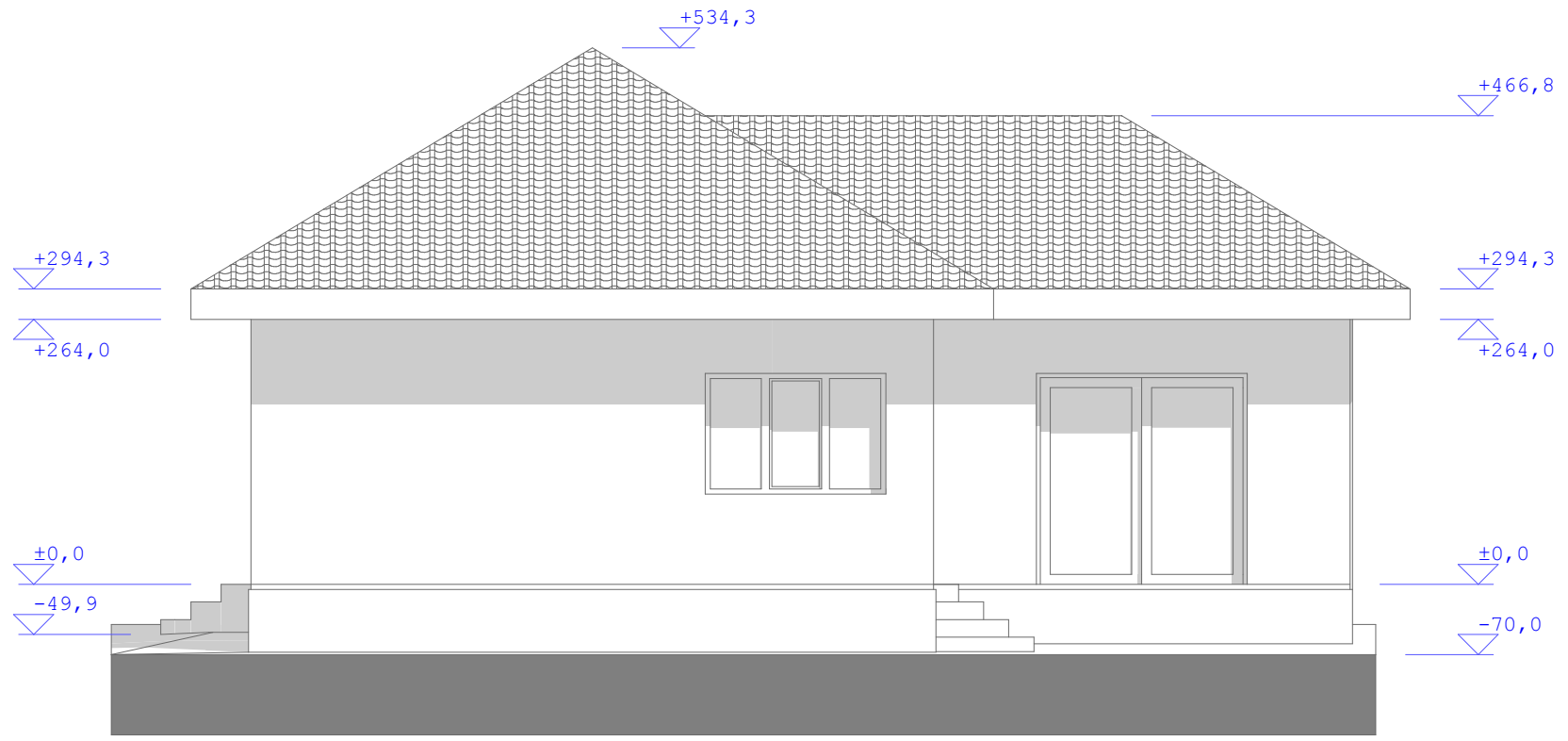
FAȚADA SUD-EST - SITUAȚIA EXISTENTĂ 1:70
